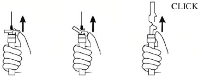
Figura 6. Cómo empujar el dispositivo de seguridad LuproLoc para que quede en el lugar
