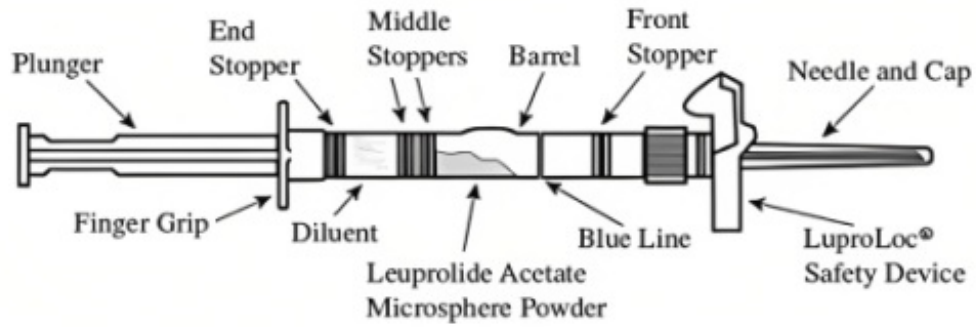
Рисунок 1. Конструкция шприца
