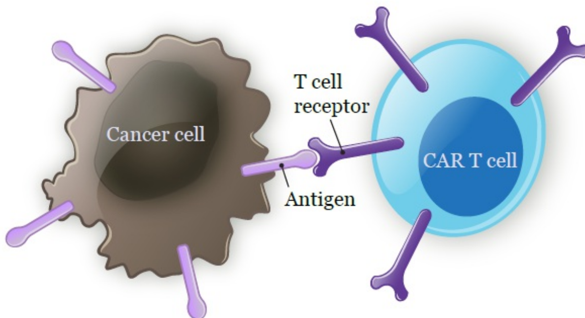
圖 2. CAR T 細胞附著在癌細胞上
